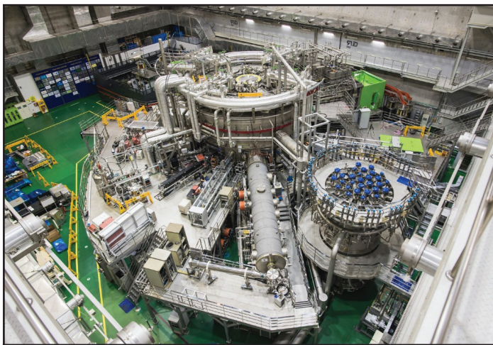
Токамак, Национален изследователски център по наука и технологии, Южна Корея
