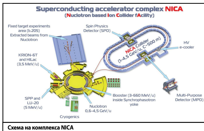
Схема на комплекса NICA
