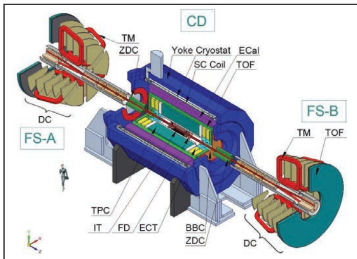
Фиг. 2. Схема на многоцелевия детектор MPD
