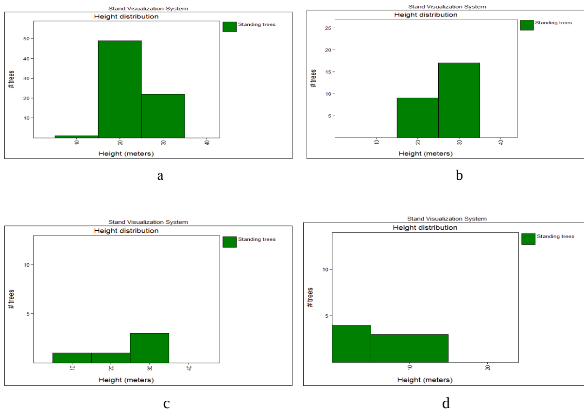
Фиг. 2. Разпределение на дърветата по височина от ОП1 ( a - Pinus sylvestris L. – бял бор) и ОП2 ( b - бял бор; c - Picea abies Karst. – смърч; d - смърчов подраст
