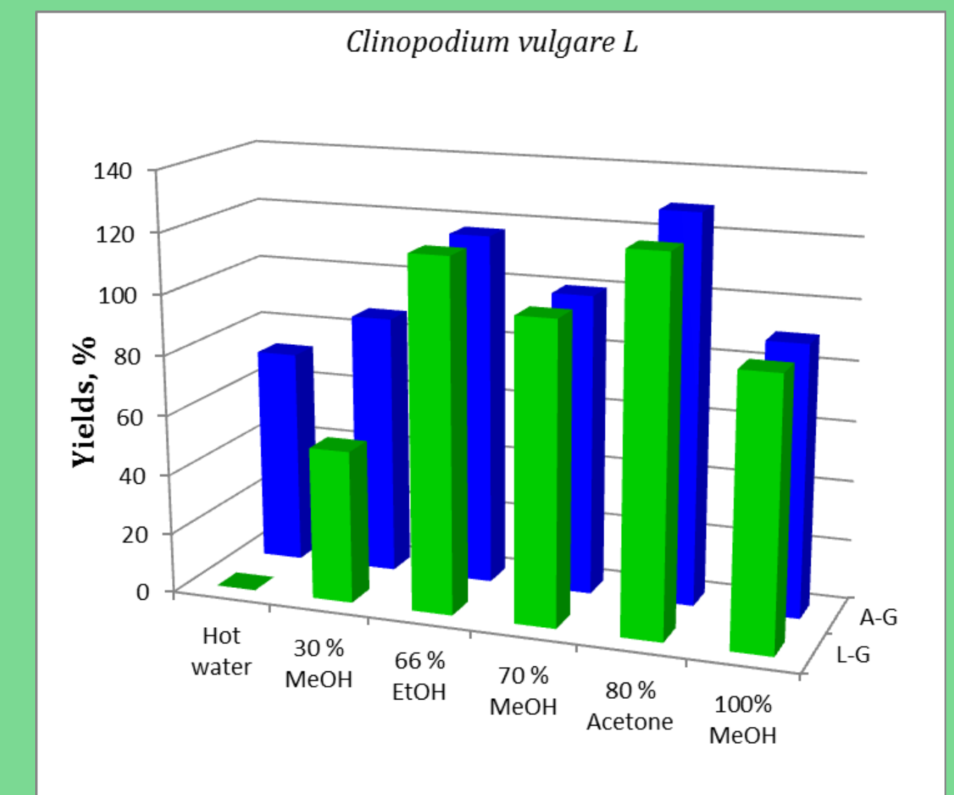
Фиг. 5. Добив на флавоноидни гликозиди (%) от Clinopodium vulgare L., получени чрез различни разтворители
