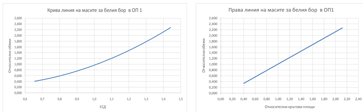
Фигура 5. Крива и права линия на масите за белия бор в ОП1 (а), белия бор (b) и смърча (с) в ОП2.
