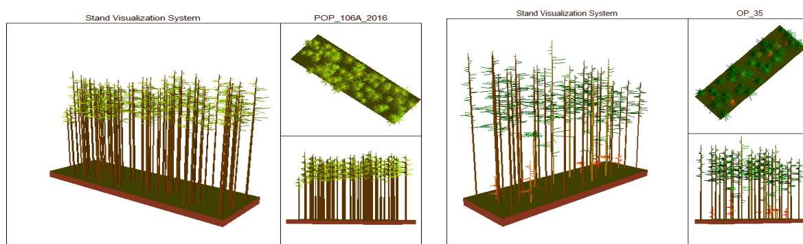
Фиг. 1. Вертикална структура на дървостойите (ОП1) – чиста белборова култура и ОП2 – смесено насаждение от бял бор и смърч
