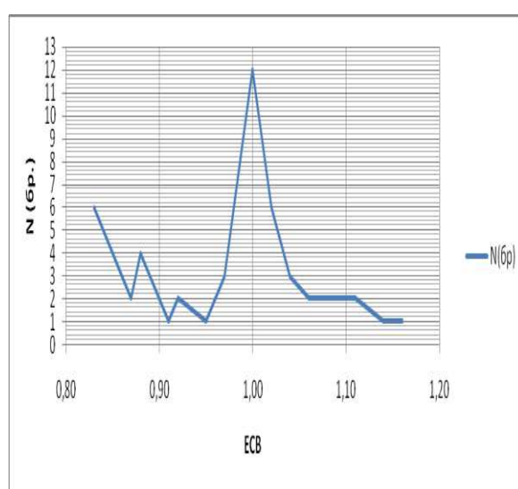
Фигура 1. Вариационни криви на разпределение на броя на дърветата от бял бор в ОП 1 (а) и от бял бор ОП2 (b) и смърч ОП2 (с) по естествени степени на височина
