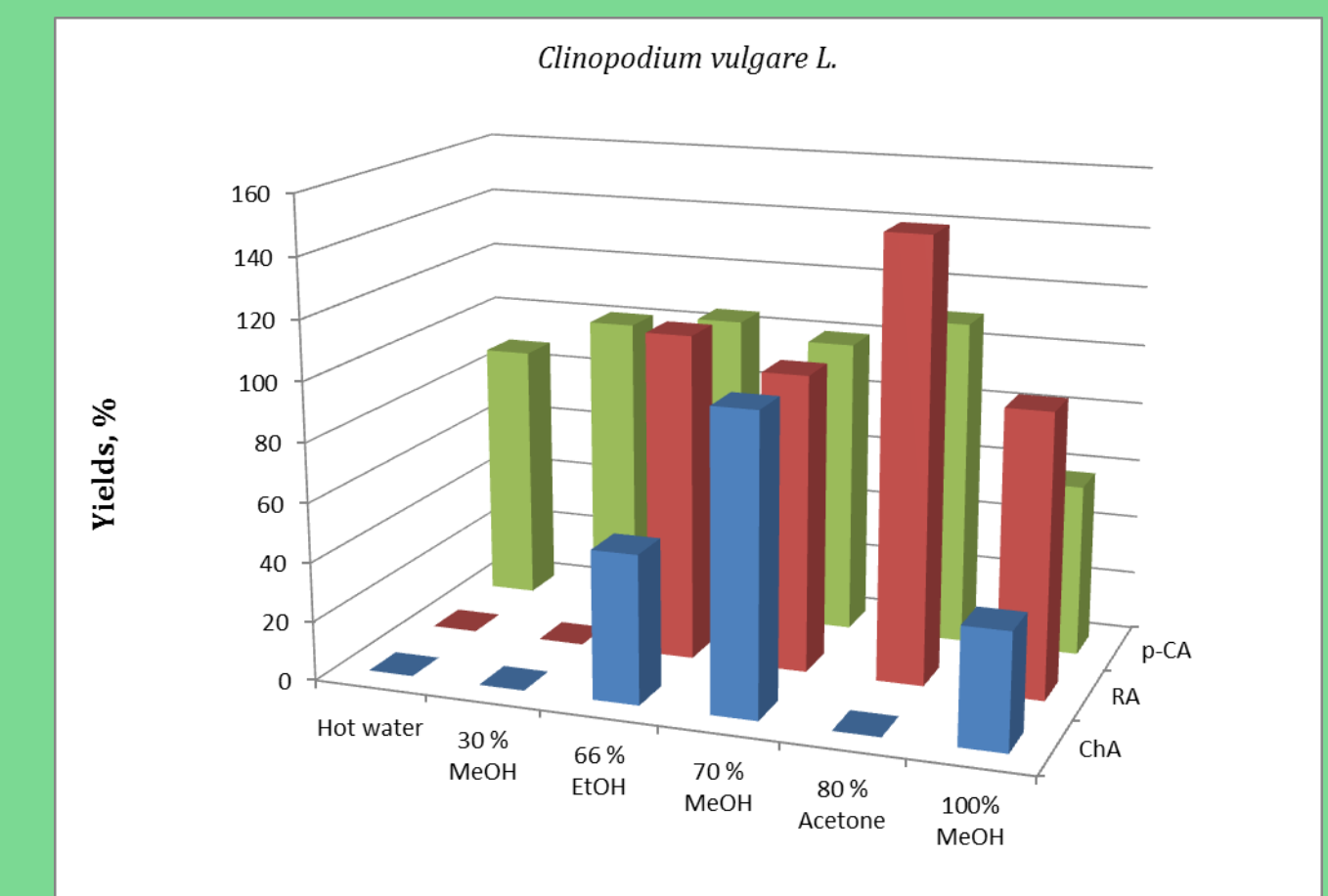
Фиг. 4. Добив на основни фенолни киселини (%) от Clinopodium vulgare L., получени чрез различни разтворители
