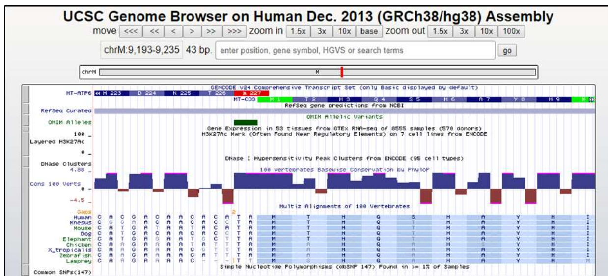
Фиг. 1 Геномна локализация на цитохром с III оксидаза (CO3) гена, показваща белтъчната секвенция. От представената схема е видно че липсват налични данни до момента в OMIM базата данни за идентифицираният от нас митохондриален вариант.
